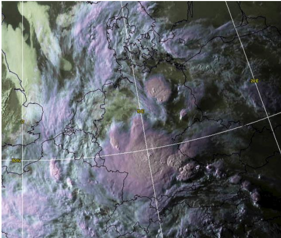
Abbildung 2: Satellitenbild MSG VIS, 29.5.2016, 18 UTC. Quelle: Eumetsat/B.J.Burton. http://www.woksat.info/wwp.html
