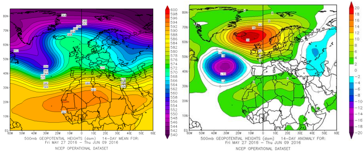
Abbildung 1: 500 hPa-Geopotential. 14-Tage-Mittelwert 27.5.-9.6.2016 (links) und Abweichung vom Mittel 1979-1995 (rechts). Bildquelle: NOAA/ESRL Physical Sciences Division, Boulder Colorado, http://www.esrl.noaa.gov/psd/
