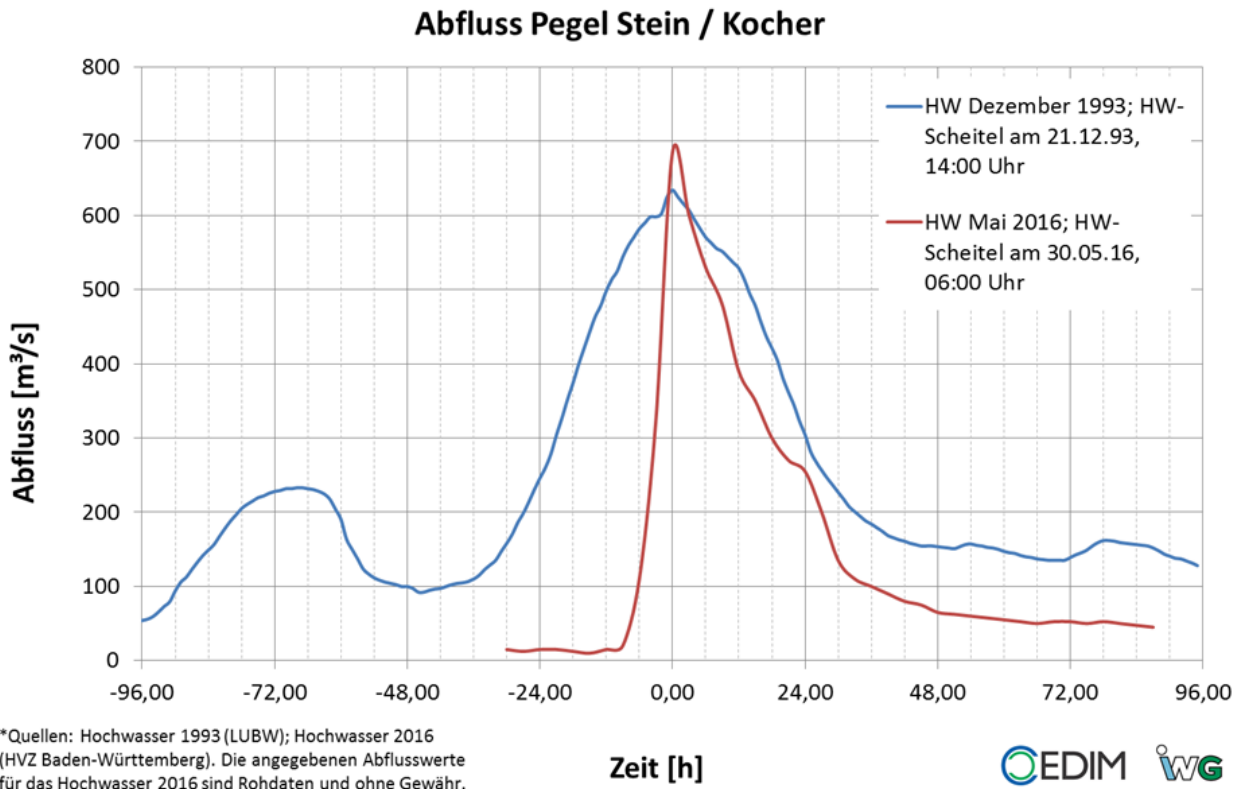
Abbildung 10: Vergleich der Abflussganglinien des aktuellen Ereignisses am Pegel Stein / Kocher mit einem Ereignis vom Dezember 1993
