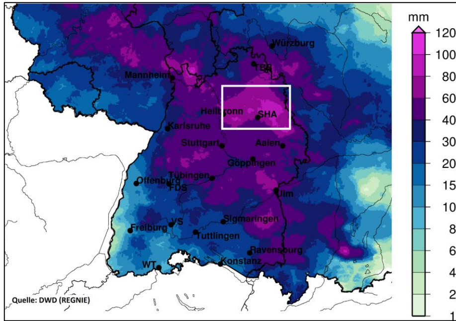
Abbildung 6: Ausschnitt aus dem REGNIE-Datensatz, 24 h Niederschlagssumme 29.5.2016 6 UTC bis 30.5.2016 6 UTC.
