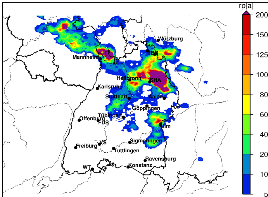
Abbildung 7: Wiederkehrperiode der 24 h Niederschlagssumme 29.5.2016 6 UTC bis 30.5.2016 6 UTC
