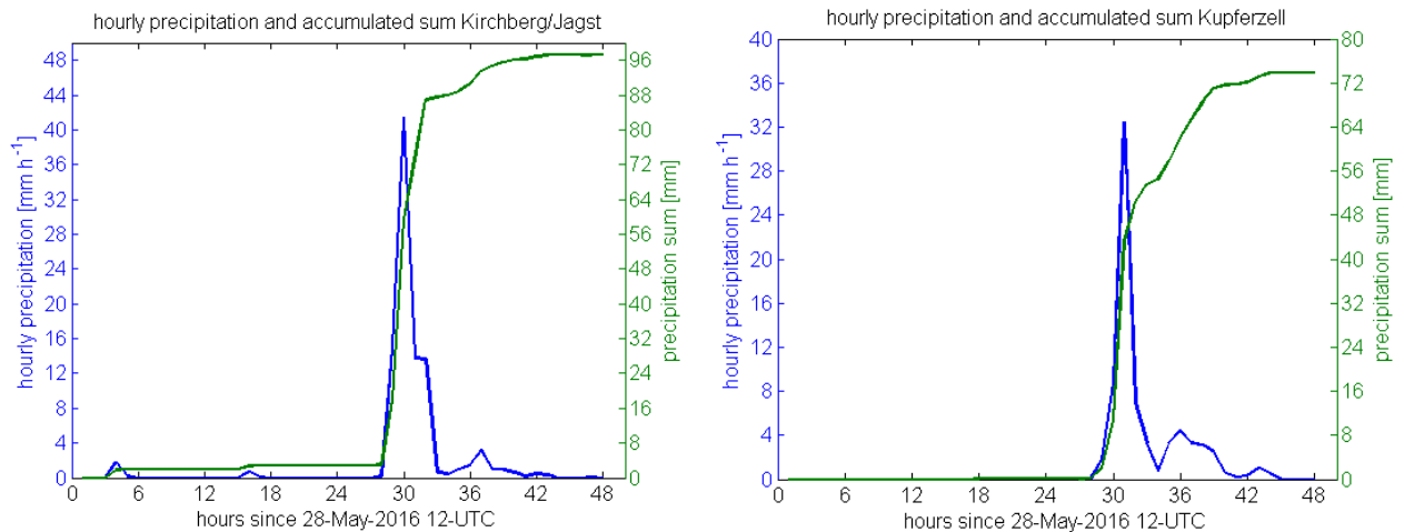
Abbildung 8: Stündliche Niederschlagswerte (blaue Kurve) der DWD-Stationen Kirchberg/Jagst (links) und Kupferzell (rechts) und akkumulierte Niederschlagssumme (grüne Kurve) für den Zeitraum 28.5.2016 12 UTC bis 30.5.2016 12 UTC.
